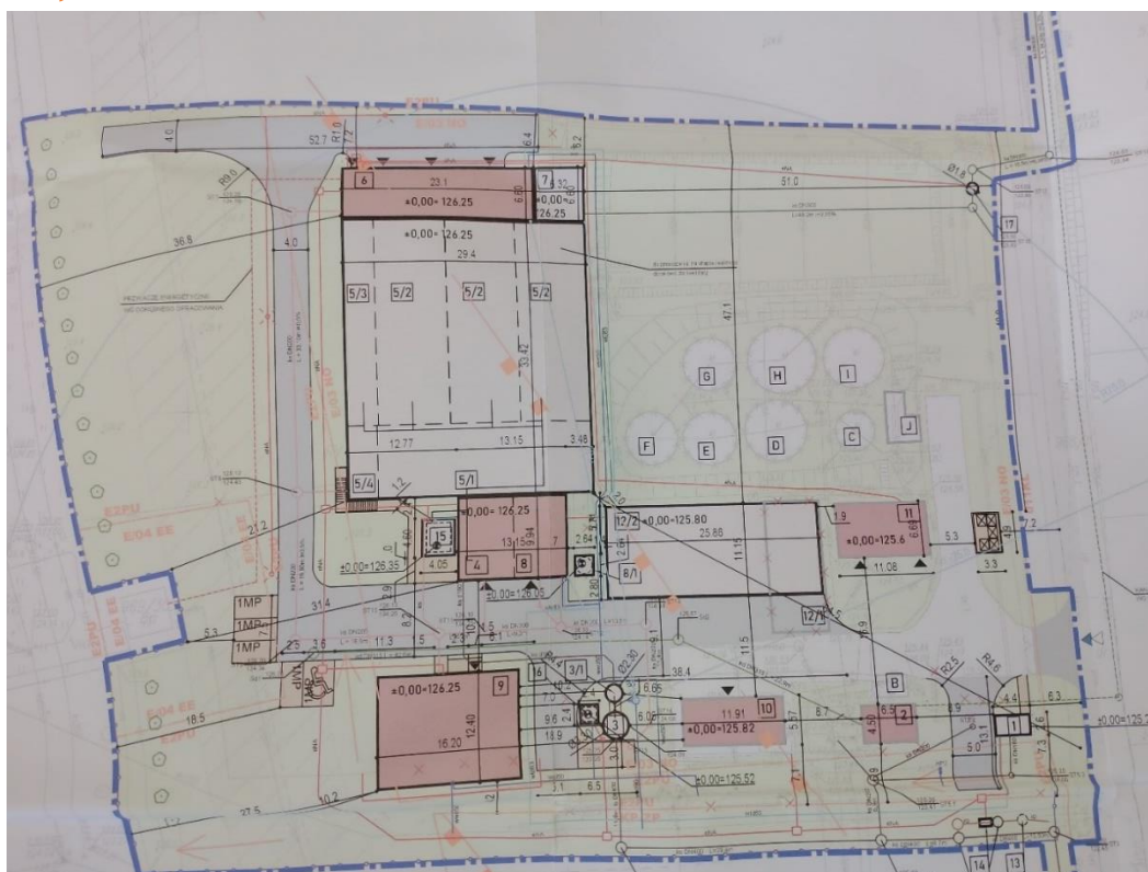
Fot. Projekt zagospodarowania terenu oczyszczalni ścieków w m. Szczuczyn
