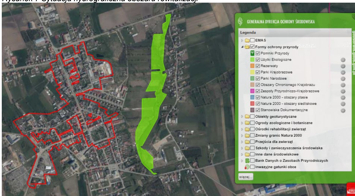
Rysunek 7 Sytuacja hydrograficzna obszaru rewitalizacji
